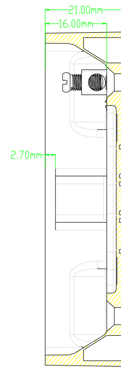
截面 A-A
